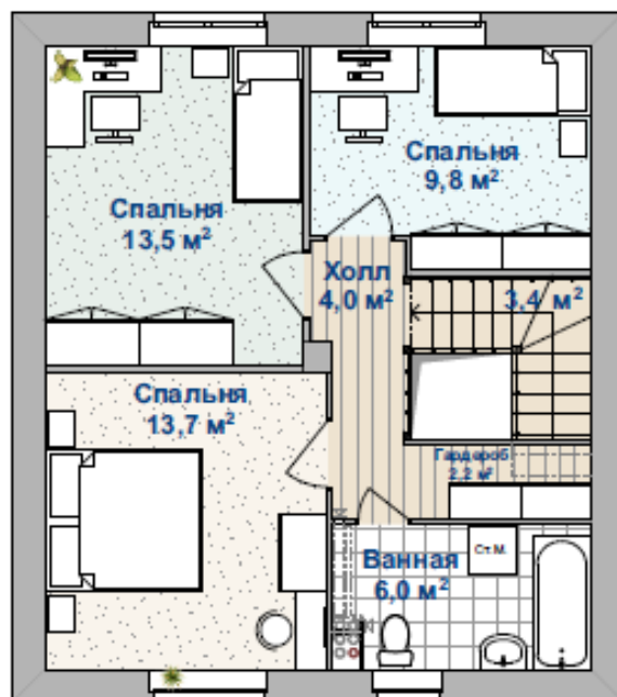
ПЛАН 2 ЭТАЖА
