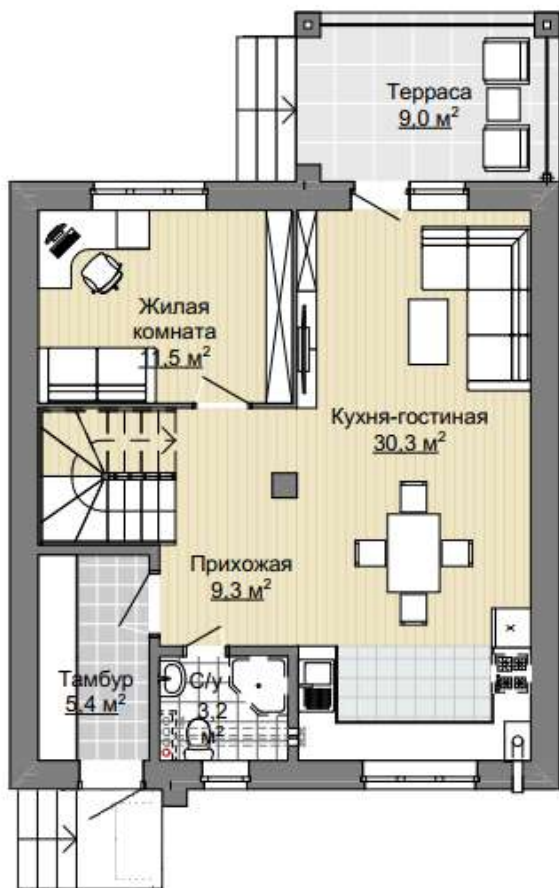
План 1-го этажа
