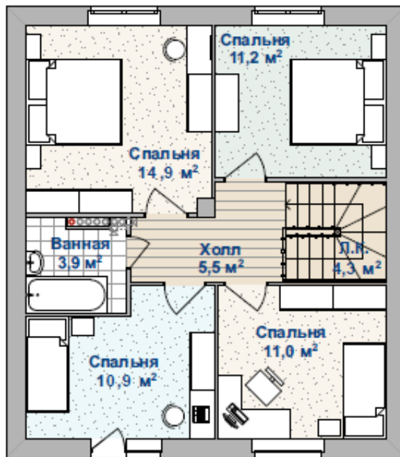
ПЛАН 2 ЭТАЖА
