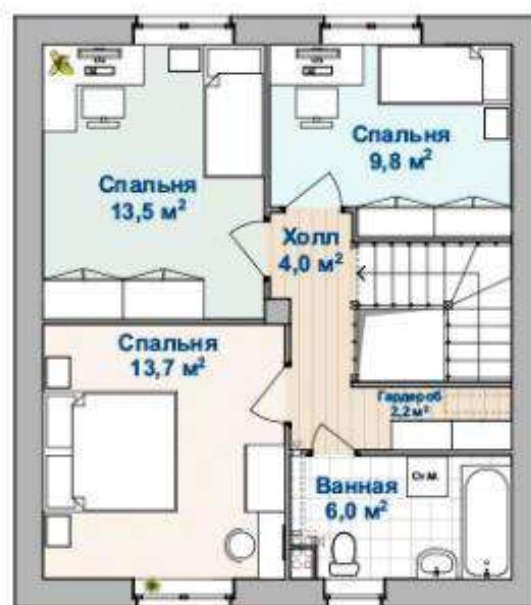
ПЛАН 2 ЭТАЖА
