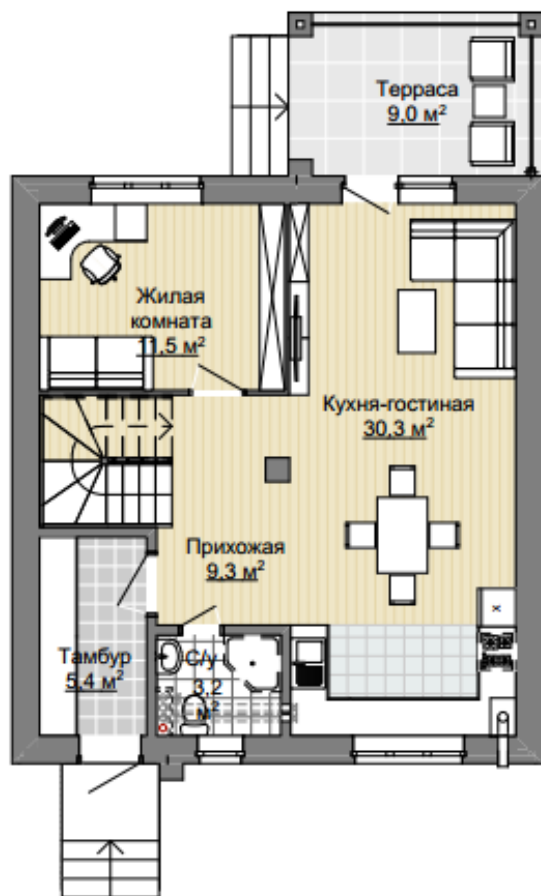
План 1-го этажа
